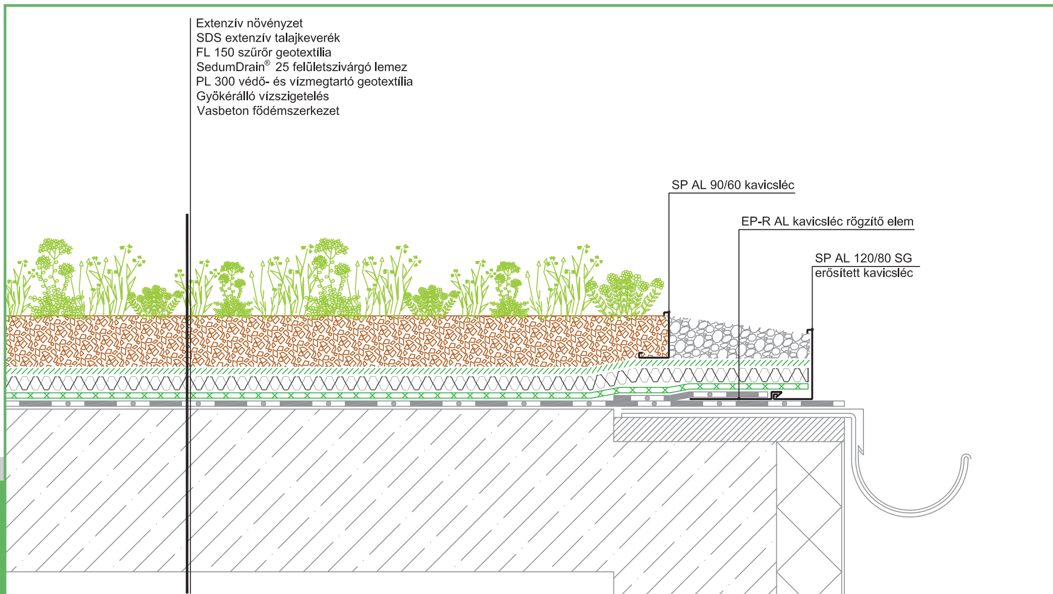
Attika nélküli tetőeresz extenzív zöldtetőn EP-R AL kavicsléc rögzítő elem
