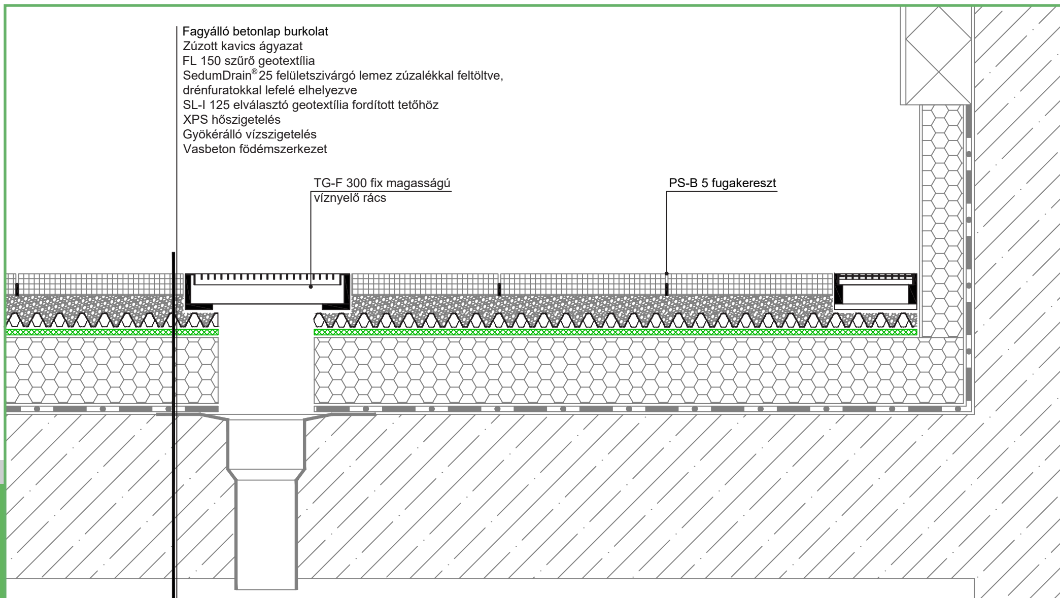
Összefolyó zöldtető teraszburkolaton 2 TG-F fix magasságú víznyelő rács
