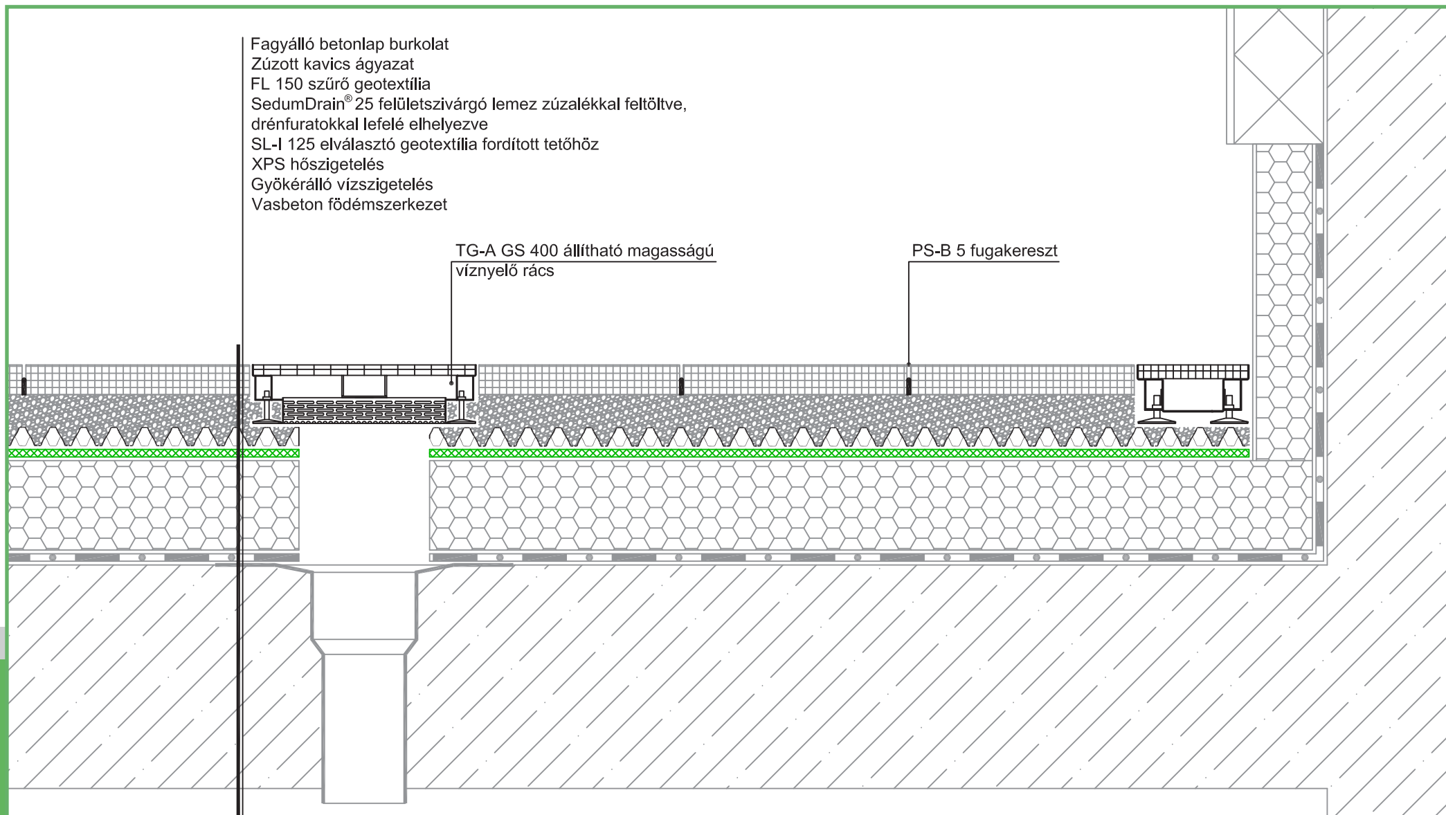
Összefolyó zöldtető teraszburkolaton 1 TG-A GS állítható magasságú víznyelő rács
