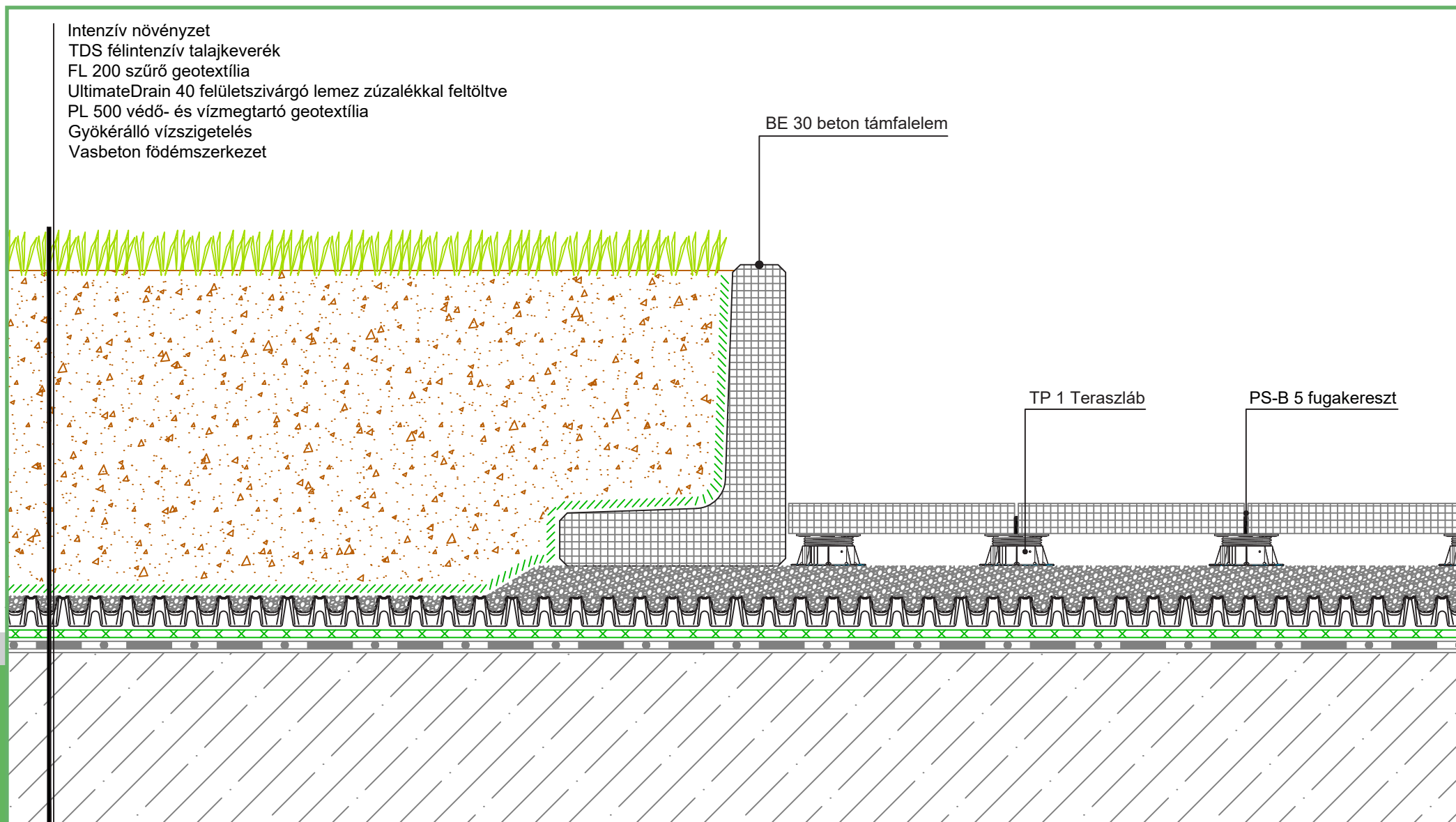
Szegélyezés intenzív zöldtetőn BE betonelem
