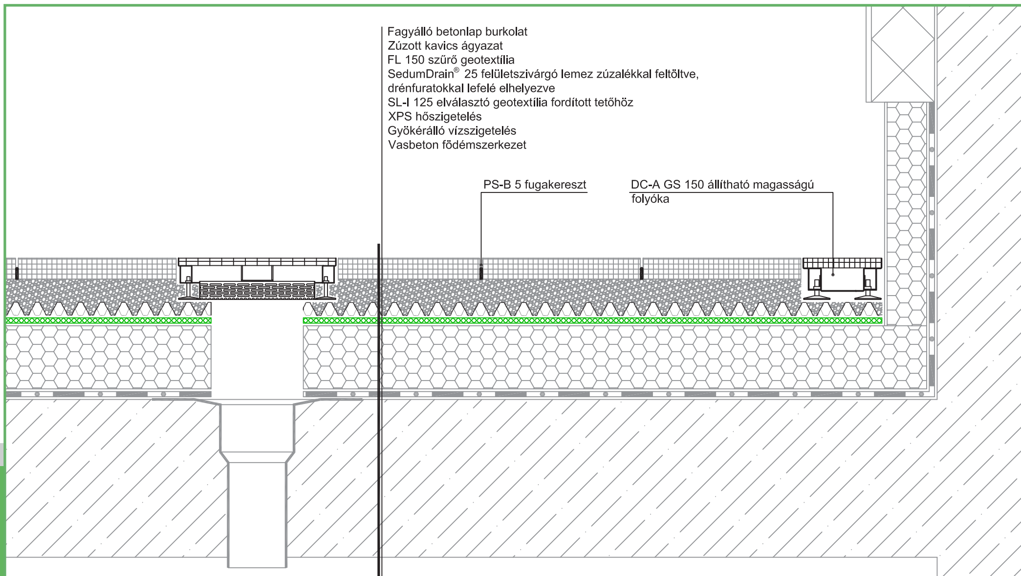
Falcsatlakozás zöldtető teraszburkolaton 1 DC-A GS állítható magasságú folyóka
